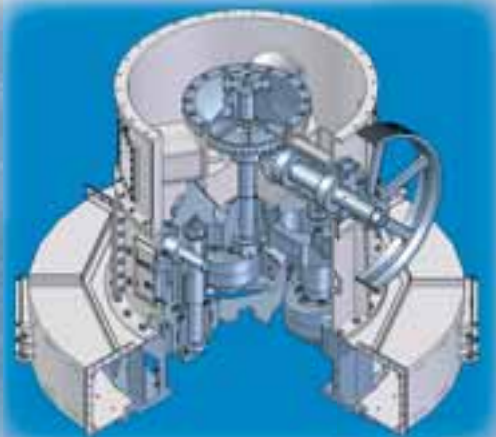
Molino pendular para coque de petróleo (por gentileza de Molaris).
